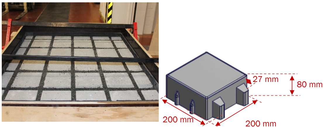
Figure 2 - Revêtement constitué et géométrie des dalles
